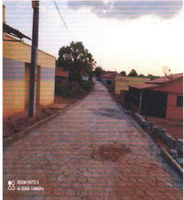
Execução de Meio fio e Pavimentação em Bloquetes (Rua Santos Dumont)
