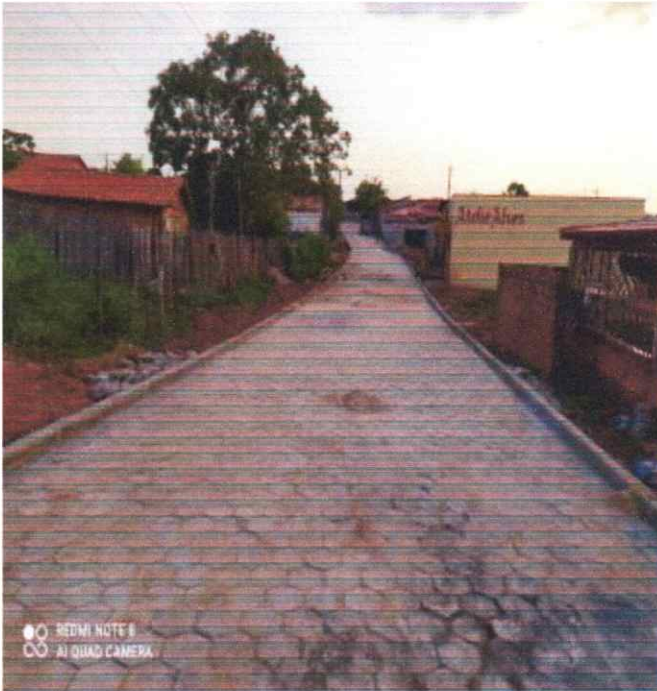
Execução de Meio fio e Pavimentação em Bloquetes (Rua Santos Dumont)
