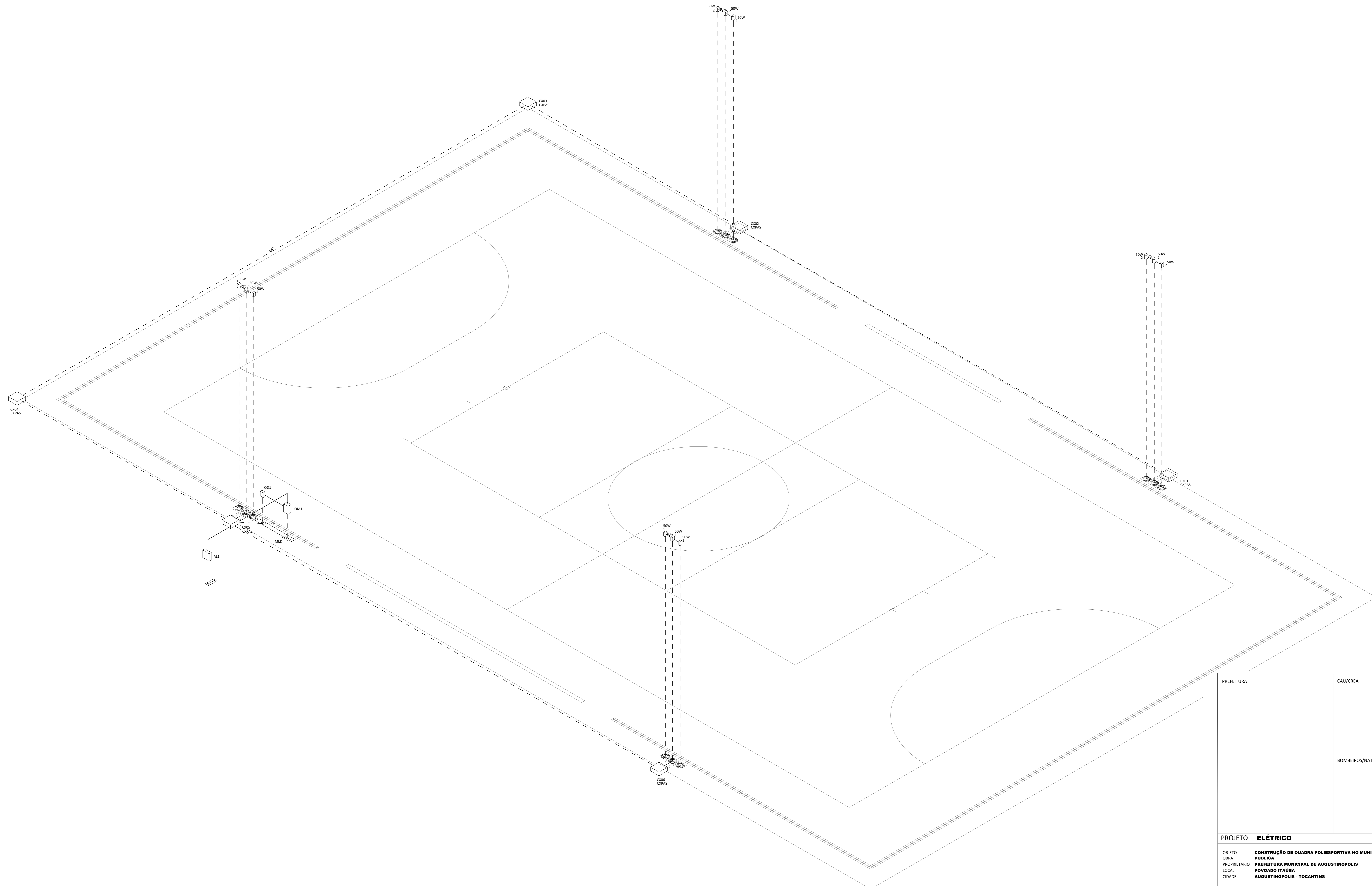
ESQUEMA ISOMÉTRICO ESCALA 1/50
