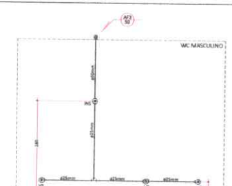
Vista AF3 Escala 1:35
