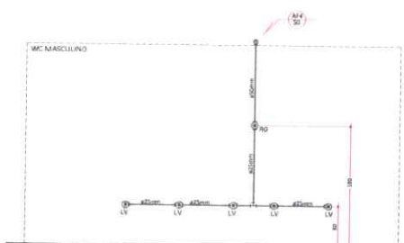
Vista AF4 Escala 1:35
