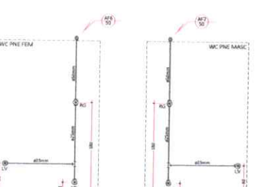
Vista AF6 Escala 1:35
