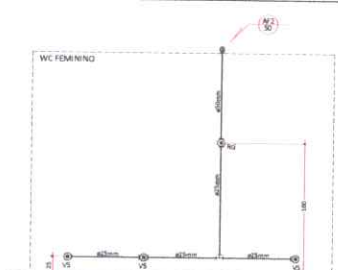
Vista AF2 Escala 1:35
