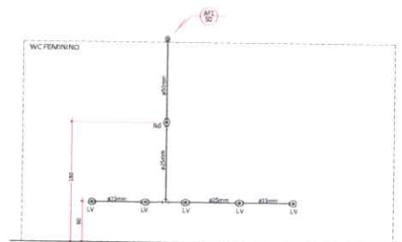
Vista AF1 Escala 1:35
