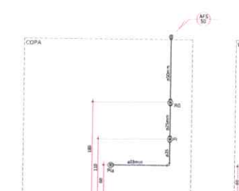
Vista AF5 Escala 1:35
