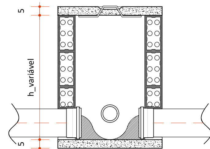
CORTE GENÉRICO CAIXA DE ESGOTO ESCALA 1/20
