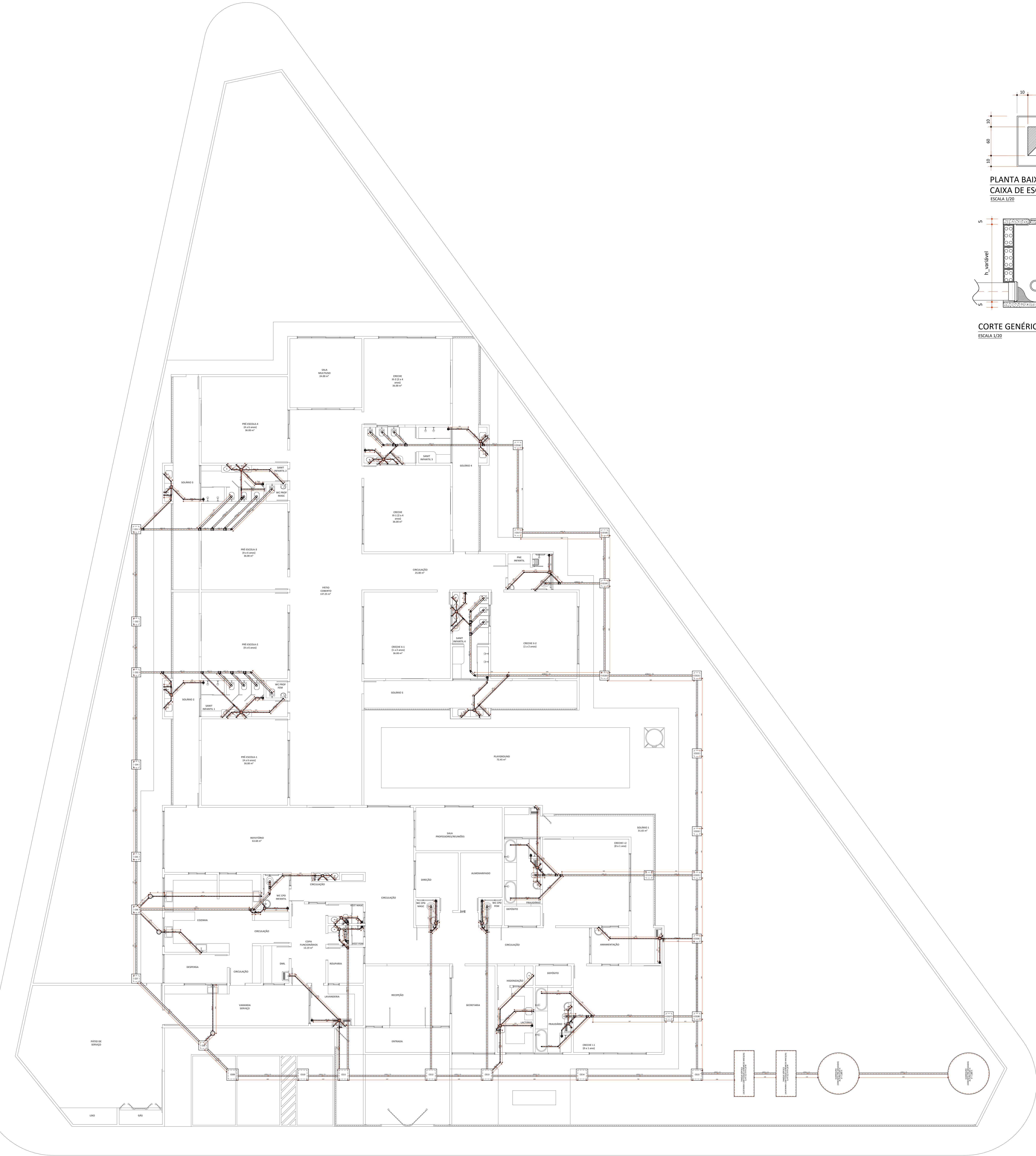
PLANTA BAIXA INSTALAÇÃO SANITÁRIA ESCALA 1/100
