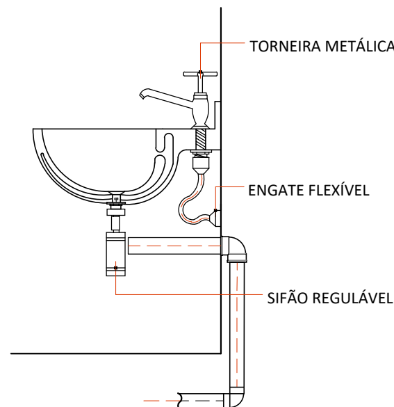
DETALHE LAVATÓRIO SEM ESCALA
