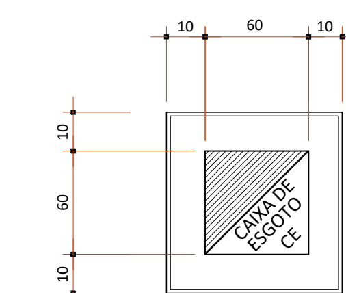
PLANTA BAIXA GENÉRICA CAIXA DE ESGOTO ESCALA 1/20
