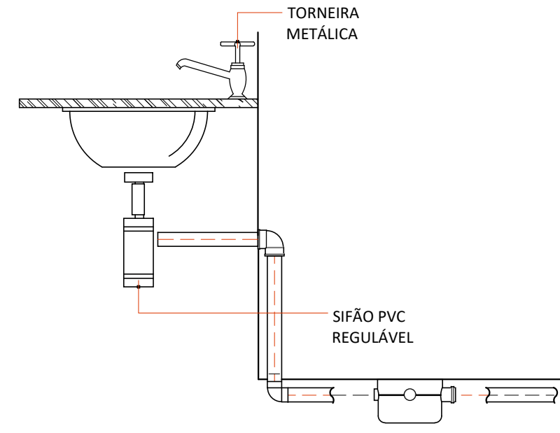
DETALHE PIA DE BANCADA SEM ESCALA
